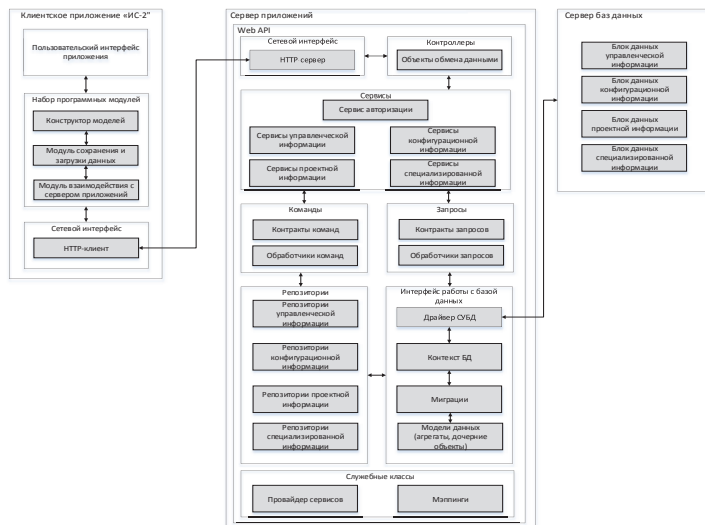
Рис. 2. Модель архитектуры «ИС - 2»
