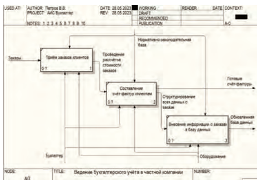
Рис. 1. Декомпозиция контекстной диаграммы «Модуль – работа с клиентами»
