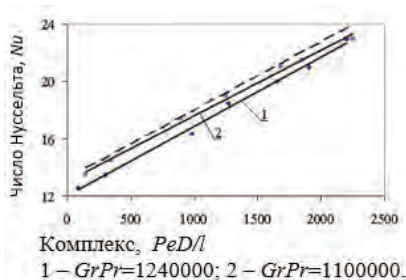
Рисунок 1 - Число Nu в гладкой круглой трубе.
