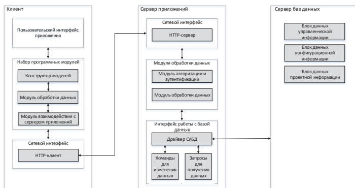
Рисунок 1. Модель типовой архитектуры CASE - системы Источник: разработано автором
