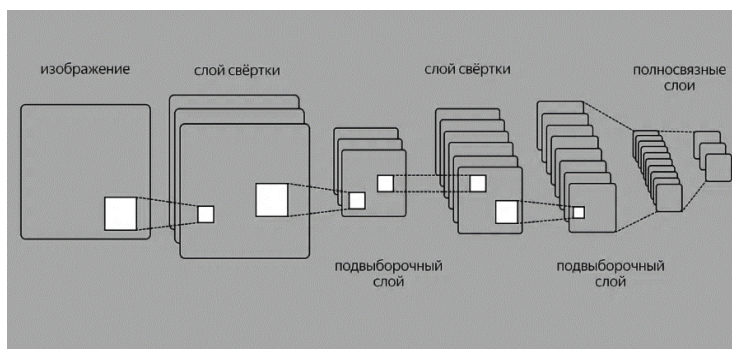
Рисунок 1 – топология сверточной нейронной сети
