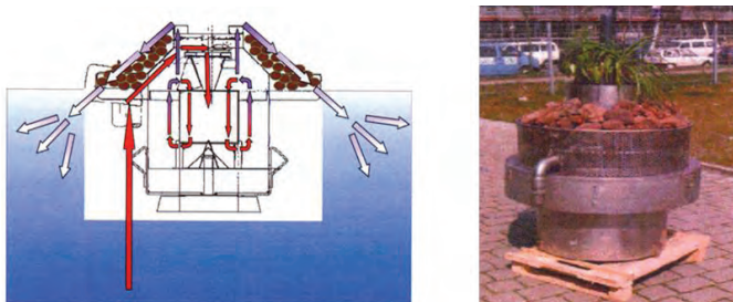
Рисунок 1. Установка «Волфиш»
