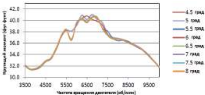
Рис. 6. Влияние угла расхождения патрубка с рестриктором на мощность двигателя
