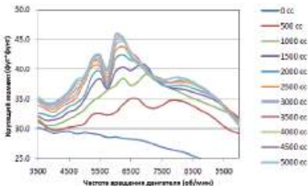
Рис. 3. Влияние объема впускного ресивера на крутящий момент
