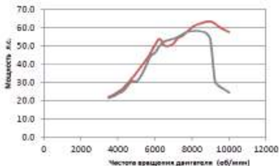
Рис. 5. Влияние формы патрубка с рестриктором на мощность двигателя
