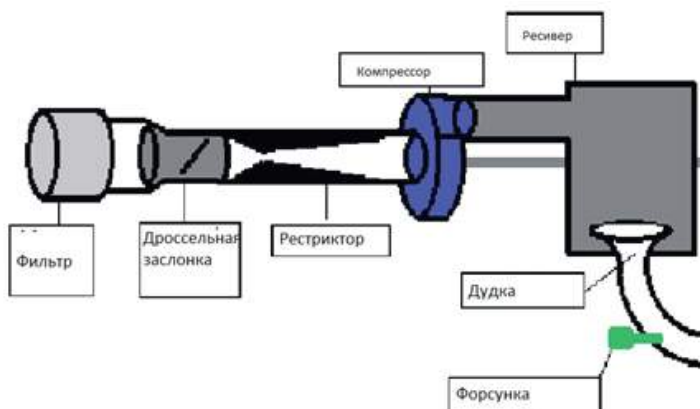
Рис. 2. Система впуска двигателя команды Формулы САИ «Cal Poly»
