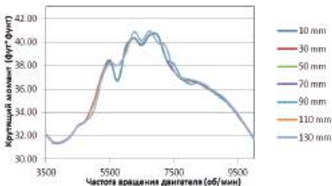
Рис. 7. Влияние длины входного патрубка на крутящий момент двигателя
